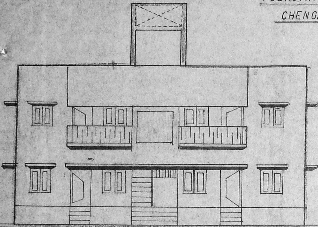
ELEVATION
